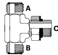
ORFSM x ORFSM x UNOM Tee
