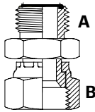
ORFSM x JICFS Adaptor
