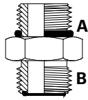
UNOM x ORFSM Nipple
