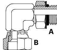
UNOM x JICFS 90° Elbow
