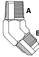
BSPTM x JICM 45° Elbow
