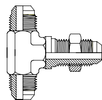
Bulkhead TEE
