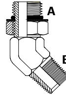
UNOM x BSPTM 45° Elbow
