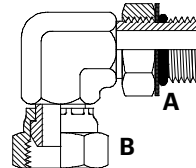
UNOM x BSPPFS 90° Elbow
