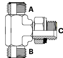
ORFSM x ORFSM x BSPPM Tee
