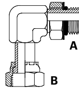
UNOM x ORFSFS 90° Elbow
