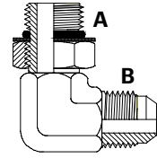
UNOM x JICM 90° Elbow
