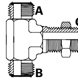
ORFSM x ORFSM x ORFSMBH Tee
