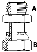
ORFSM x ORFSFS Adaptor
