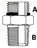
UNOM x BSPTM Nipple
