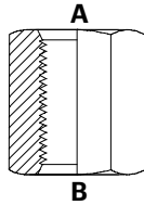
UNOF x UNOF Socket
