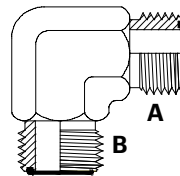
ORFSM x ORFSM 90° Elbow
