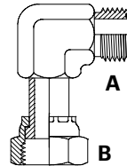
ORFSM x ORFSFS 90° Elbow
