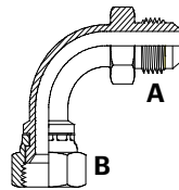
JICM x JICFS 90° Bend
