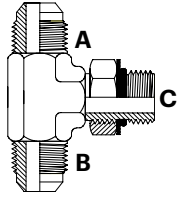
JICM x JICM x UNOM Tee
