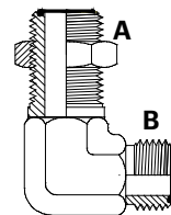
ORFSBH x ORFSM 90° Elbow
