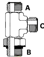
ORFSM x UNOM x ORFSM Tee
