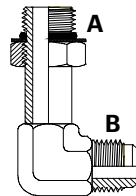
UNOM x JICM EXT 90° Bend
