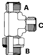
ORFSM x BSPPM x ORFSM Tee
